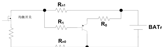
图 3：均衡原理示意图
