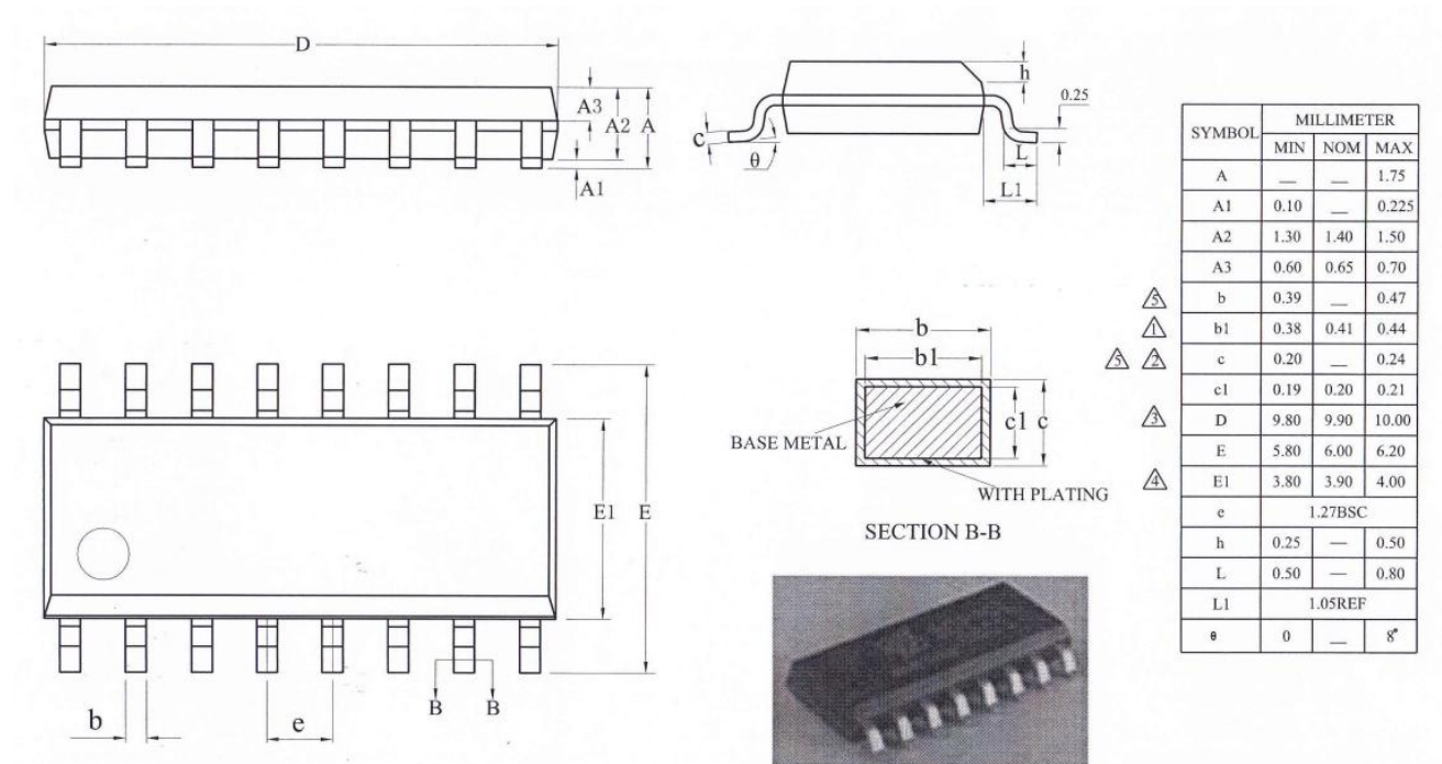
图 14: IP3265 SOP16 封装外形尺寸图
